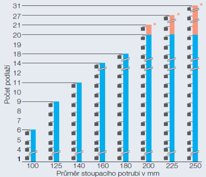
Montáž 1 ventilátoru na podlaží při plánovaném objemovém průtoku 60 m 3 /h a současném provozu všech ventilátorů.
