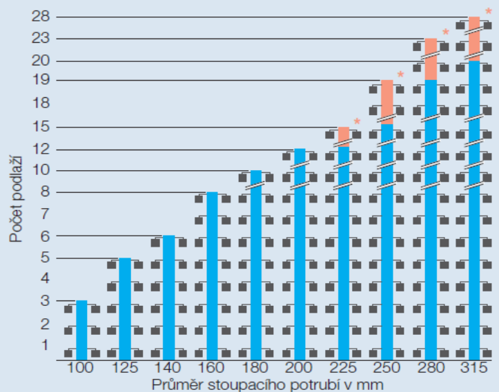
Montáž 2 ventilátorů na podlaží při plánovaném objemovém průtoku 60 m 3 /h a současném provozu všech ventilátorů.
