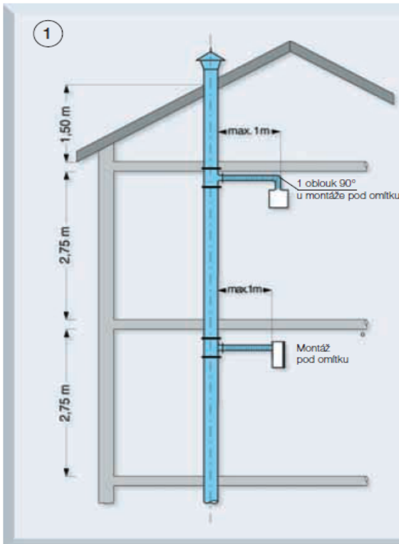
Montáž 1 ventilátoru na podlaží při plánovaném objemovém průtoku 60 m 3 /h a současném provozu všech ventilátorů.
