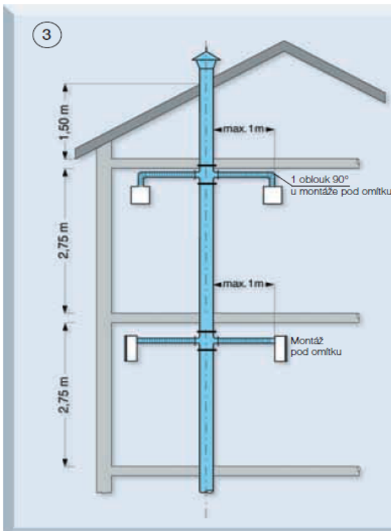
Montáž 2 ventilátorů na podlaží při plánovaném objemovém průtoku 60 m 3 /h a současném provozu všech ventilátorů.
